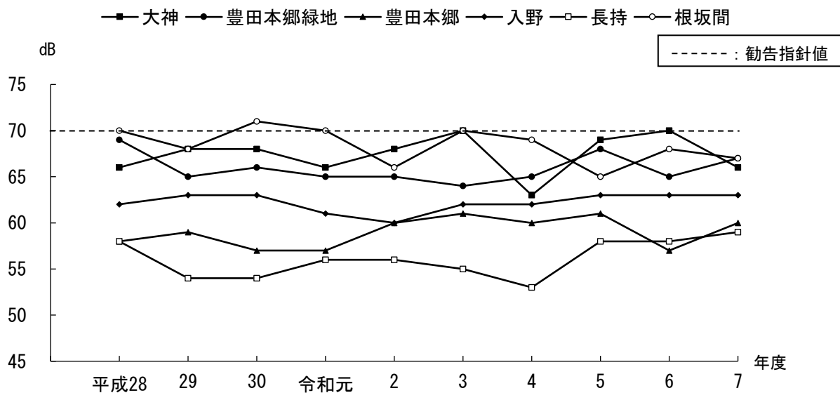
図3-8 新幹線鉄道振動測定結果経年変化
