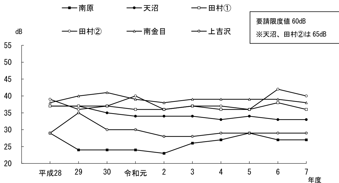
図3-5 自動車振動測定結果経年変化（夜間）
