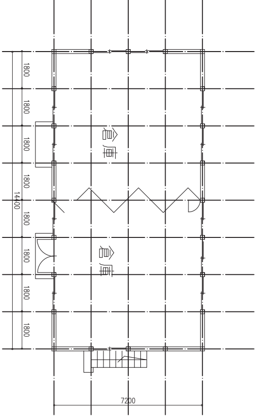
2階平面図
