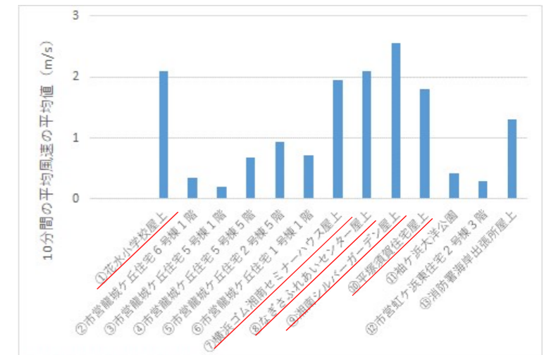
図5：各調査地点の10分間平均風速の平均値
