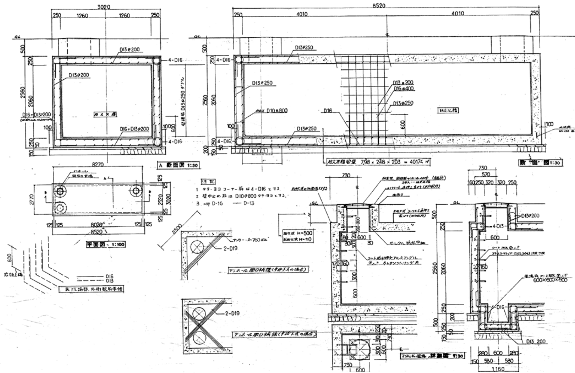
防火水槽 平面図 断面図
