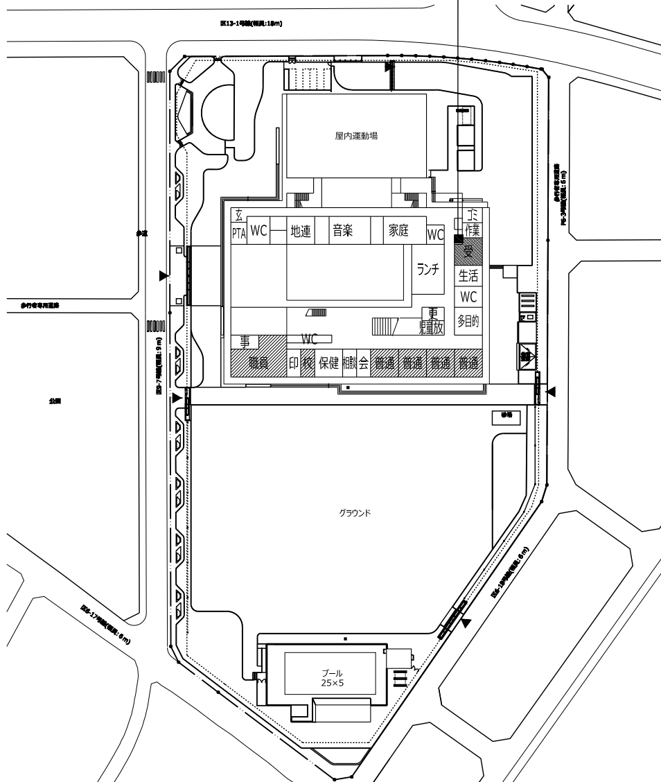
配置図兼1階平面図
