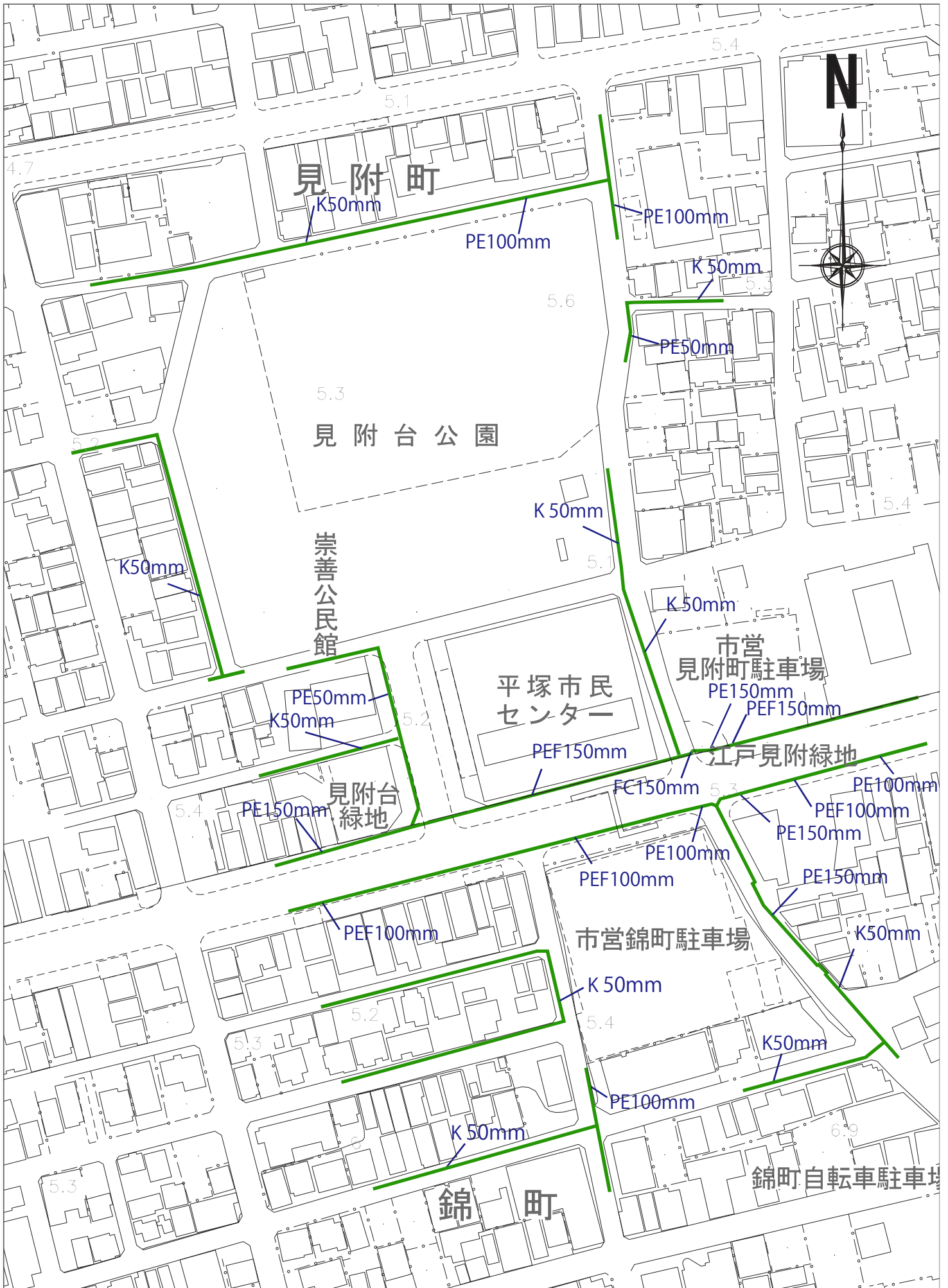
事業対象地周辺の埋設管の概要
